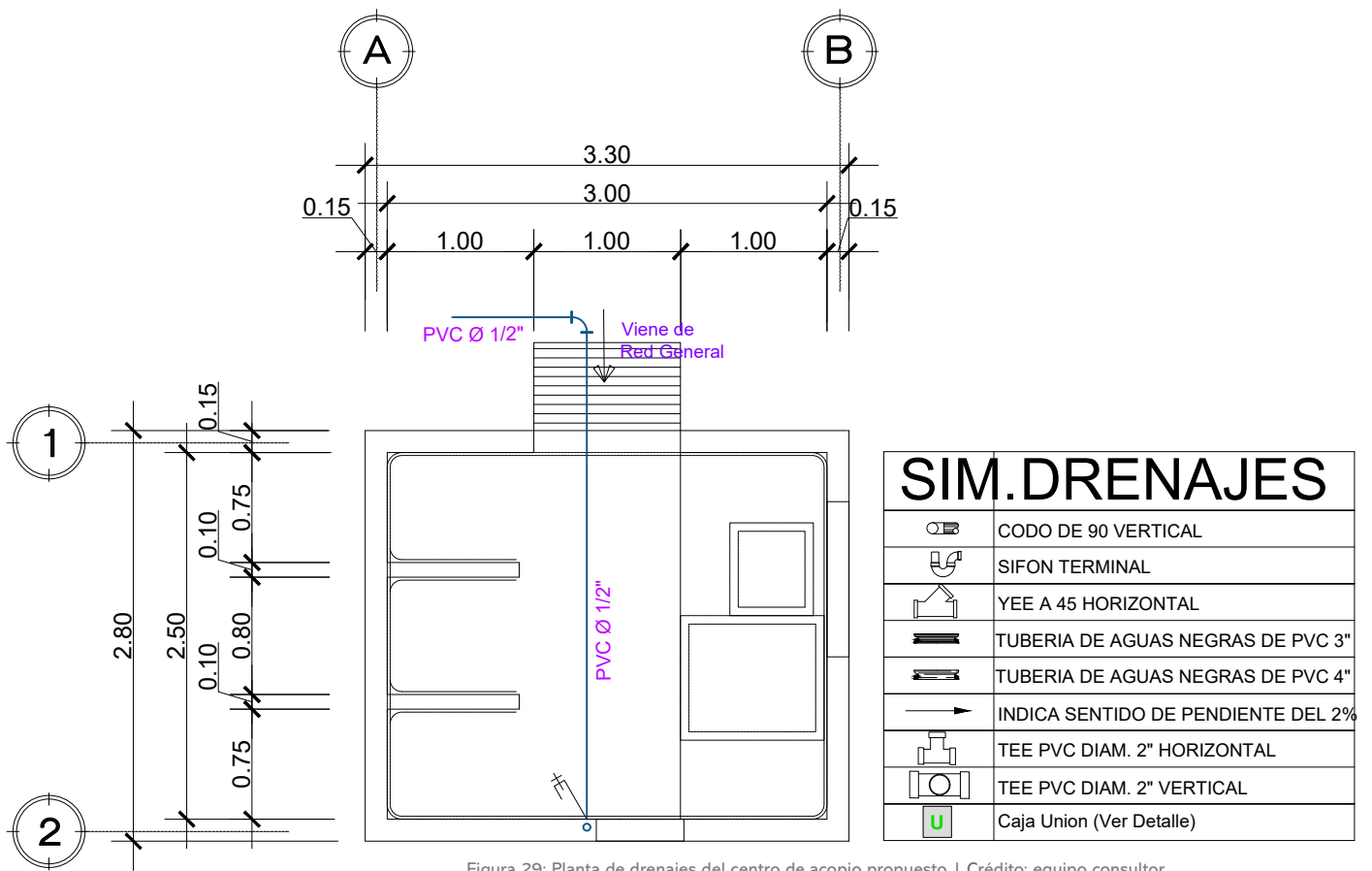
Figura 29: Planta de drenajes del centro de acopio propuesto | Crédito: equipo consultor.
