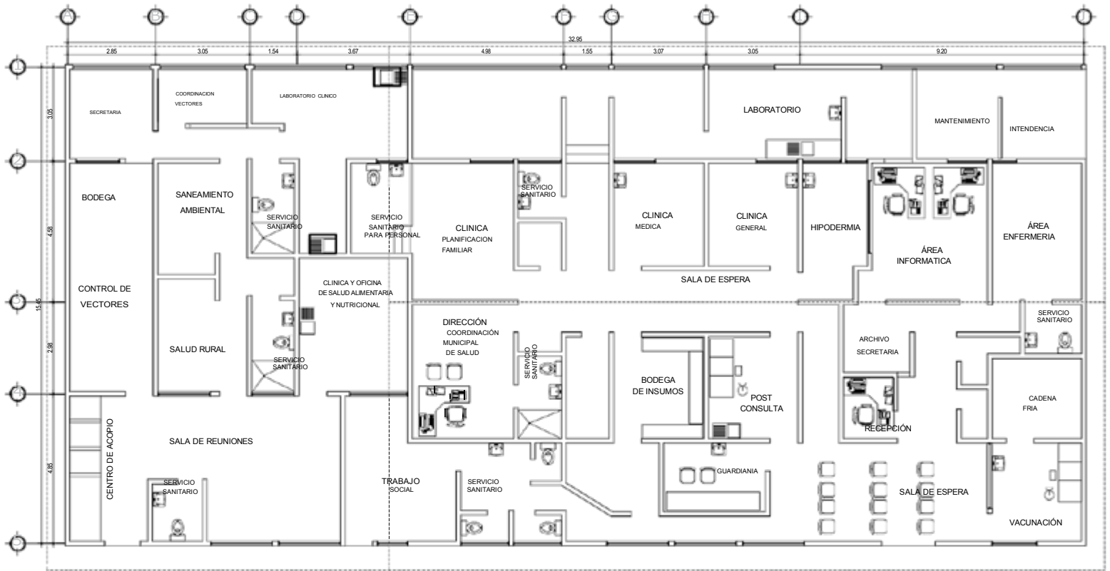
Figura 6: Plano del Centro de salud Santa Cruz Barillas | Crédito: equipo consultor.
