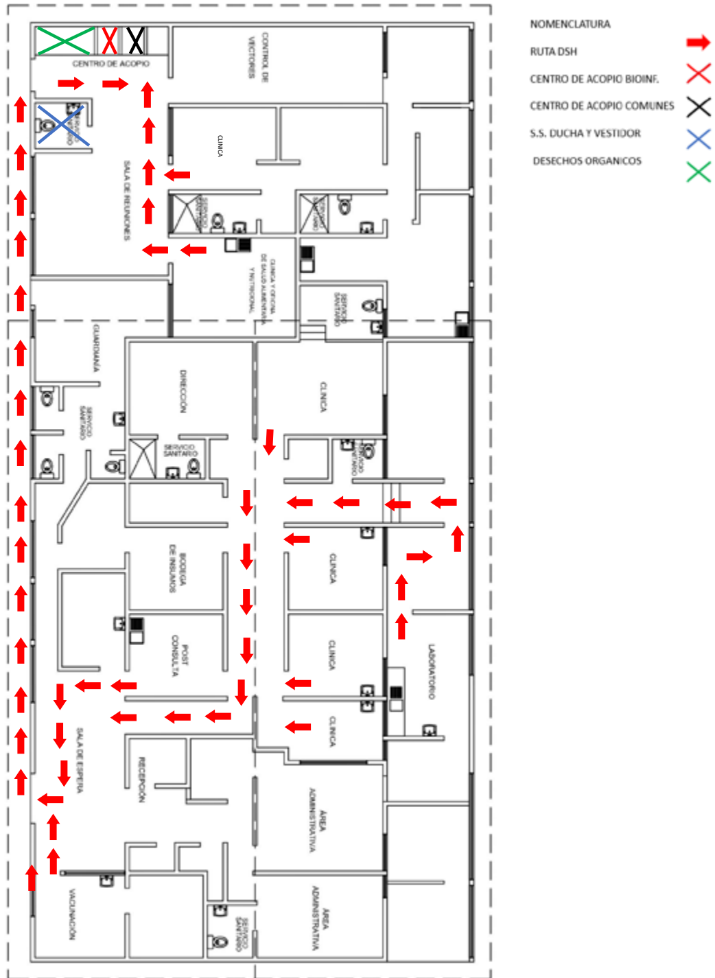
Figura 59: Plano del Centro de salud Santa Cruz Barillas | Crédito: equipo consultor.
