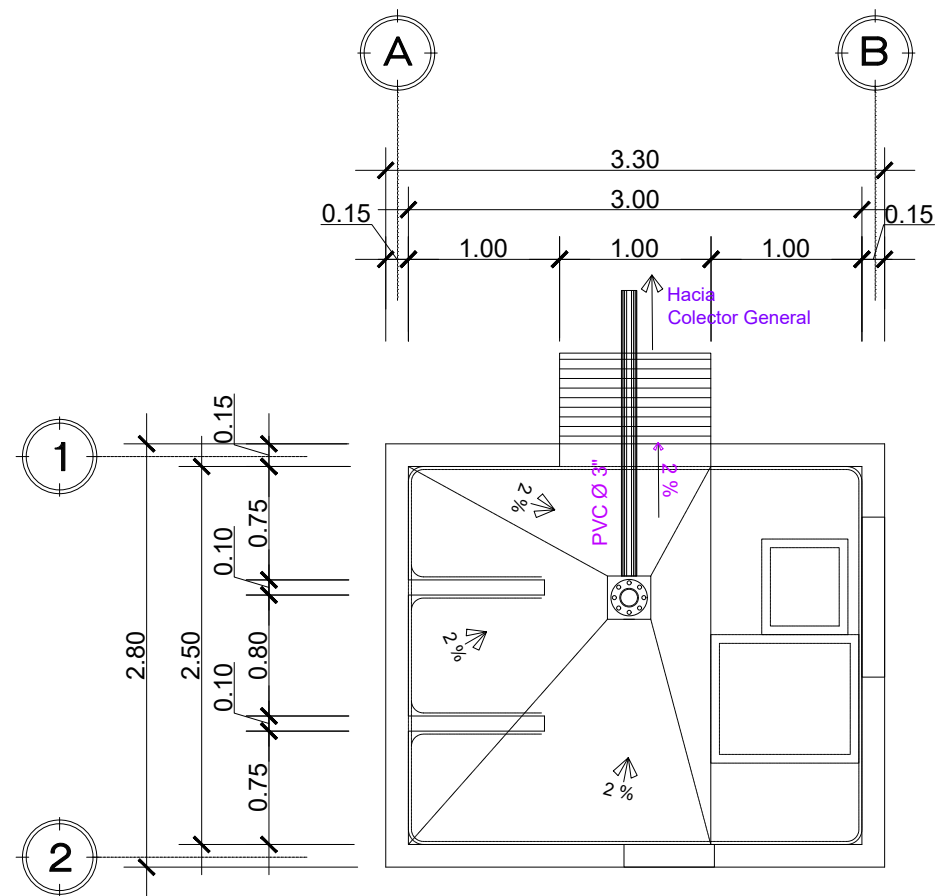
Figura 33: Planta hidráulica del centro de acopio propuesto | Crédito: equipo consultor.
