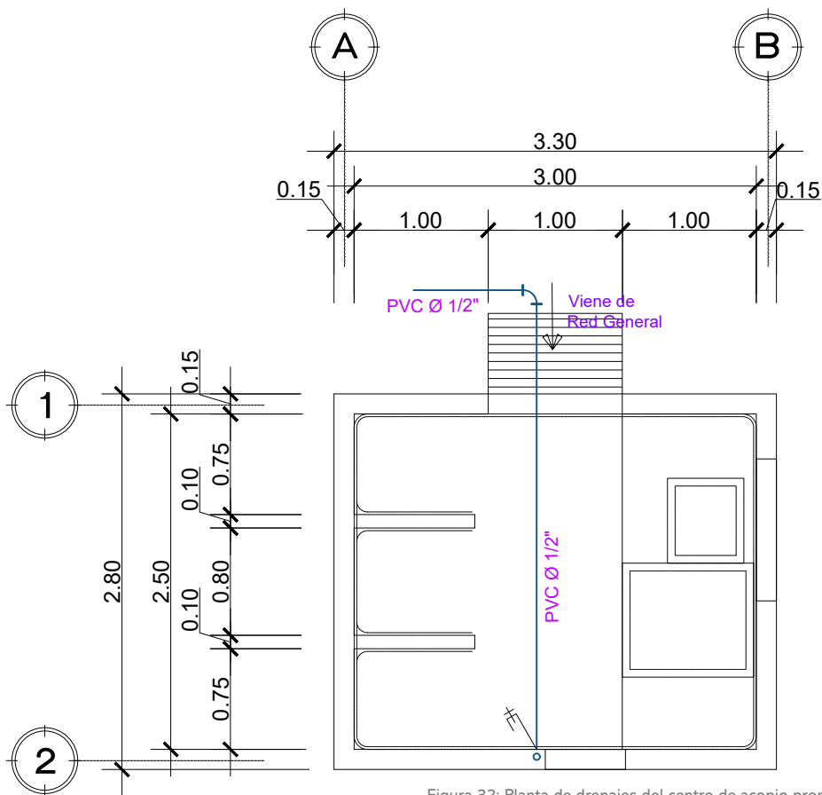
Figura 32: Planta de drenajes del centro de acopio propuesto | Crédito: equipo consultor.
