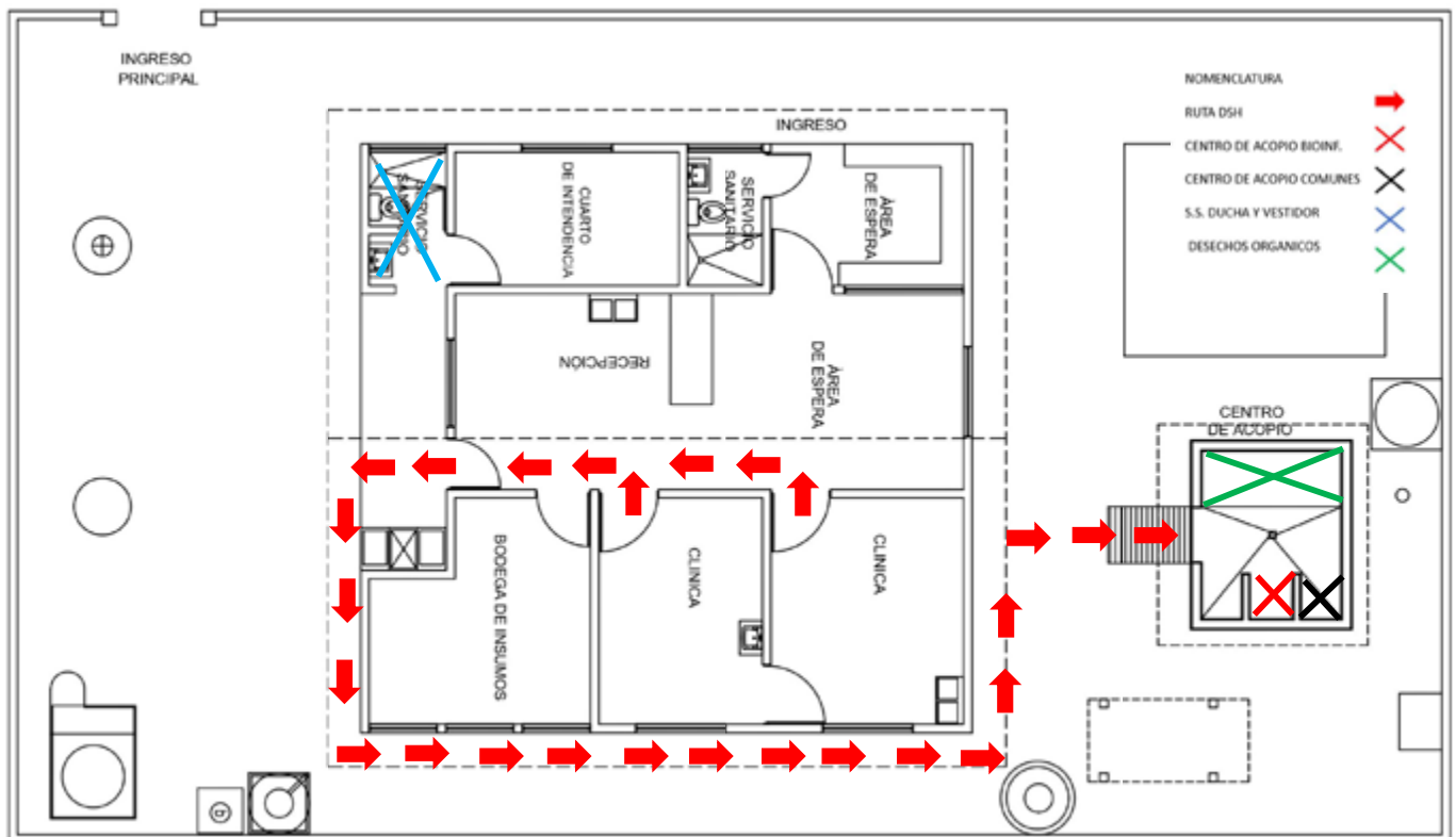
Figura 63: Plano del Puesto de salud Xoxlac | Crédito: equipo consultor.
