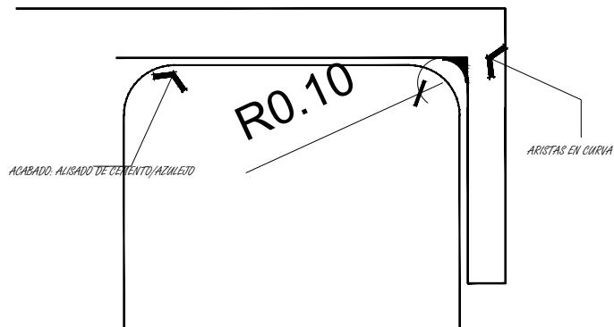
Figura 35: Detalle arista del centro de acopio propuesto, énfasis en curvas, (escala: 125) | Crédito: equipo consultor.
