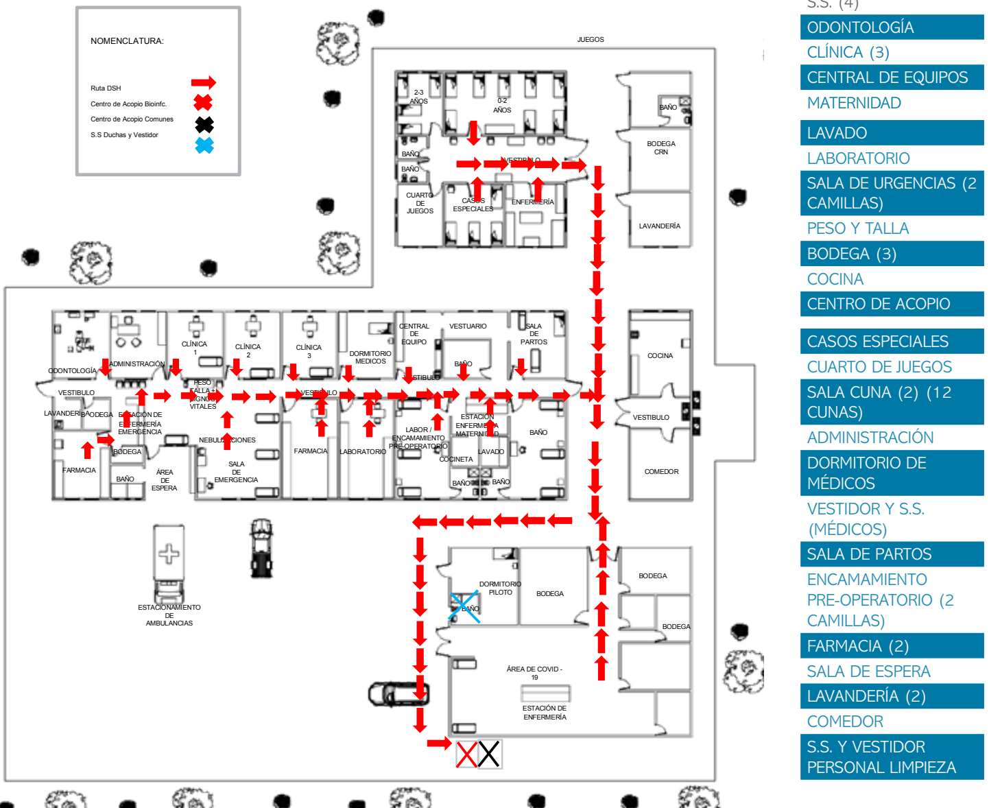
Figura 5: Plano del Centro de atención permanente Jocotán | Crédito: equipo consultor.
