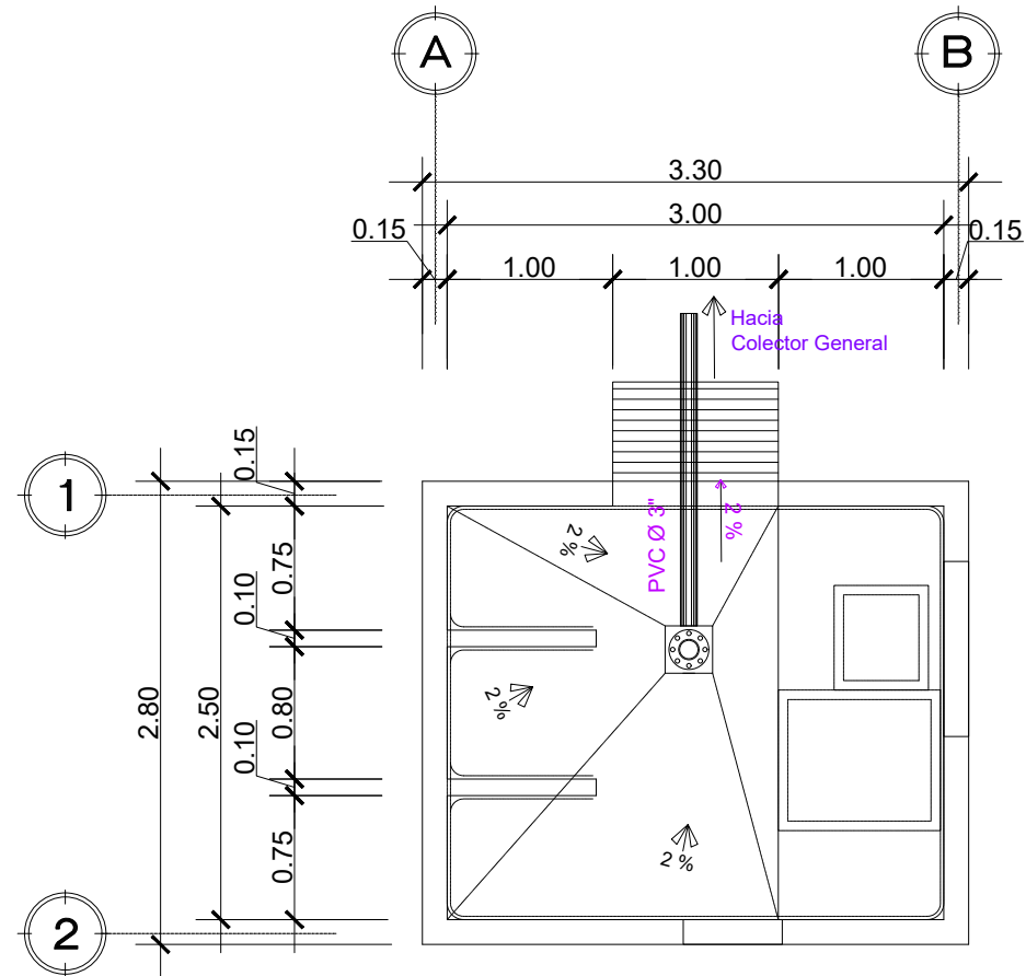
Figura 32: Planta hidráulica del centro de acopio propuesto | Crédito: equipo consultor.
