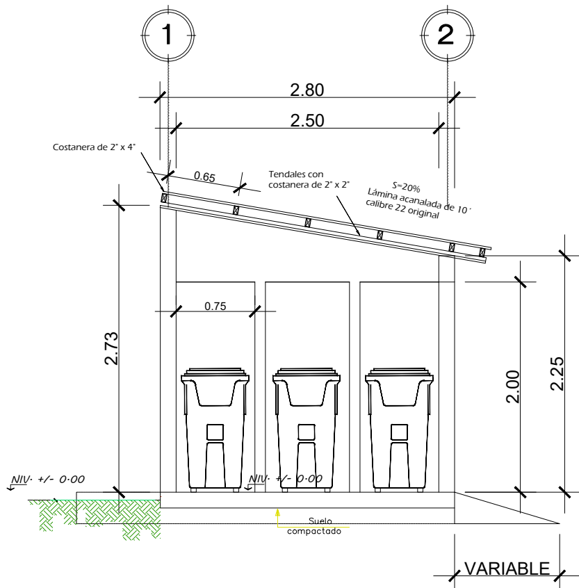
Figura 29: Sección transversal del centro de acopio propuesto | Crédito: equipo consultor.
