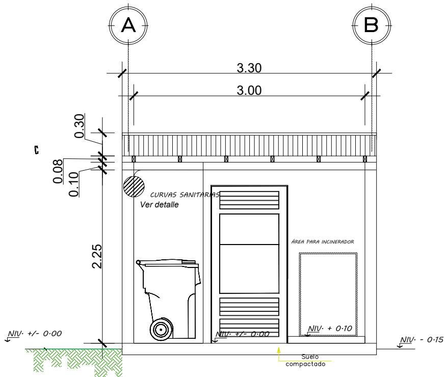
Figura 30: Sección longitudinal del centro de acopio propuesto | Crédito: equipo consultor.
