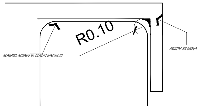
Figura 34: Detalle arista del centro de acopio propuesto, énfasis en curvas, (escala: 125) | Crédito: equipo consultor.
