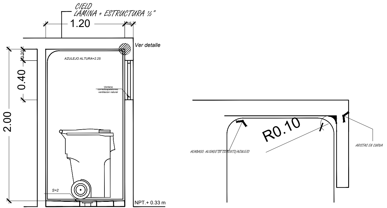
Figura 31: Detalle arista del centro de acopio propuesto (escala: 125) y detalle arista del centro de acopio propuesto, énfasis en curvas, (escala: 125) | Crédito: equipo consultor | Crédito: equipo consultor.
