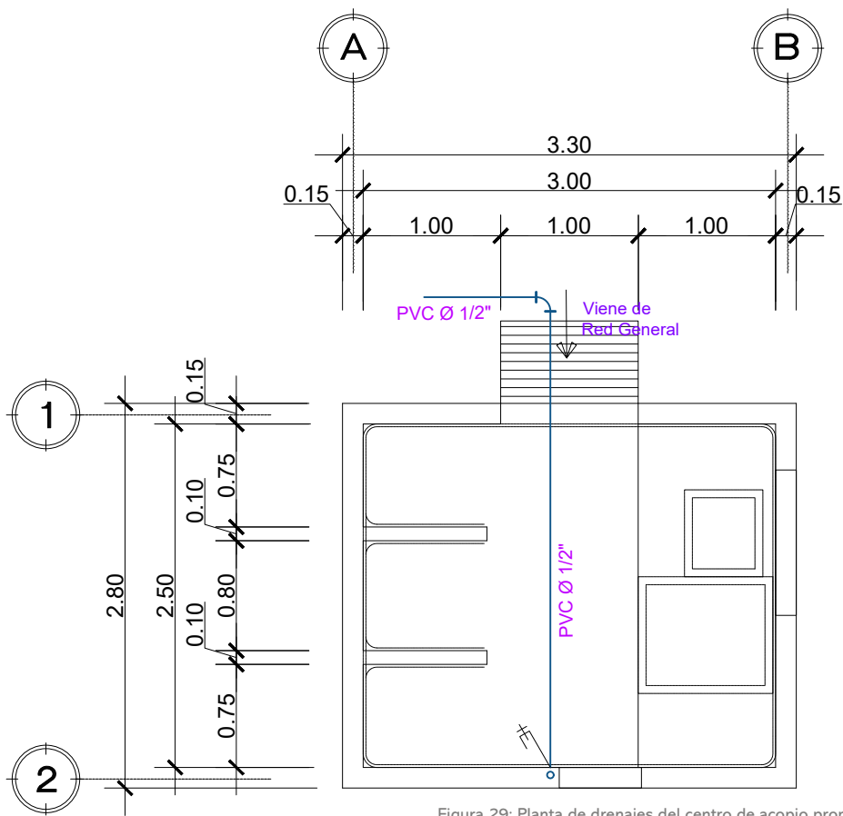
Figura 29: Planta de drenajes del centro de acopio propuesto | Crédito: equipo consultor.
