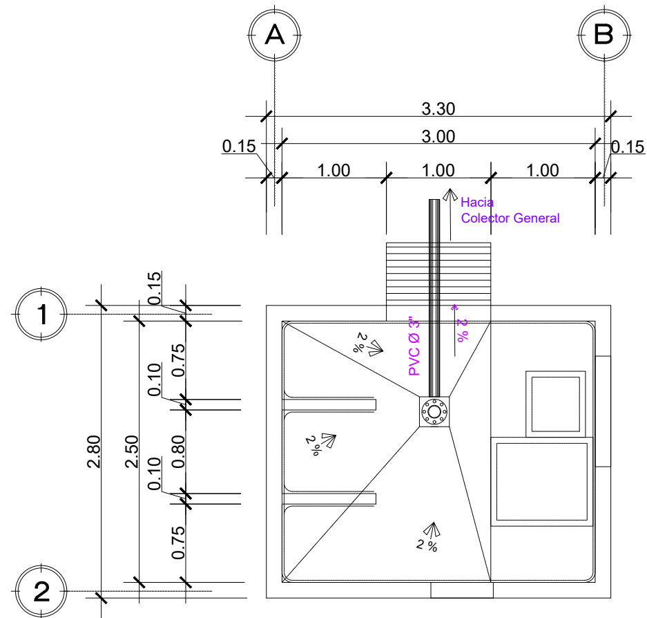
Figura 30: Planta hidráulica del centro de acopio propuesto | Crédito: equipo consultor.
