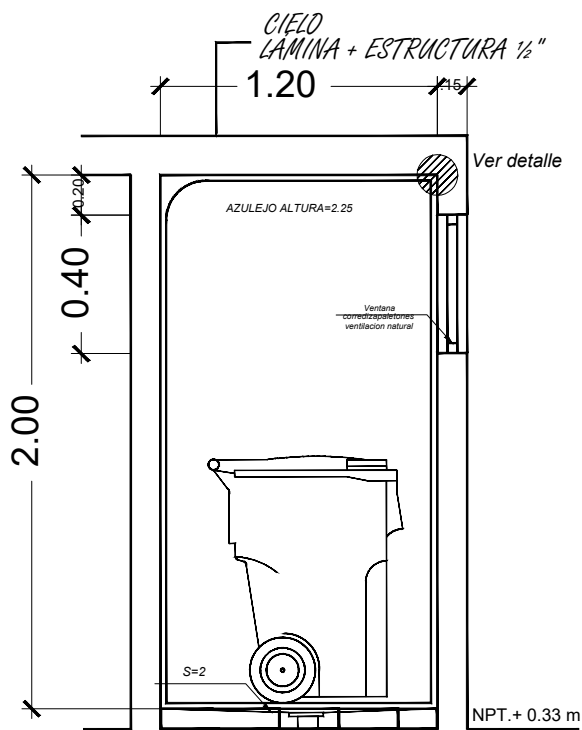
Figura 31: Detalle arista del centro de acopio propuesto (escala: 125) | Crédito: equipo consultor.
