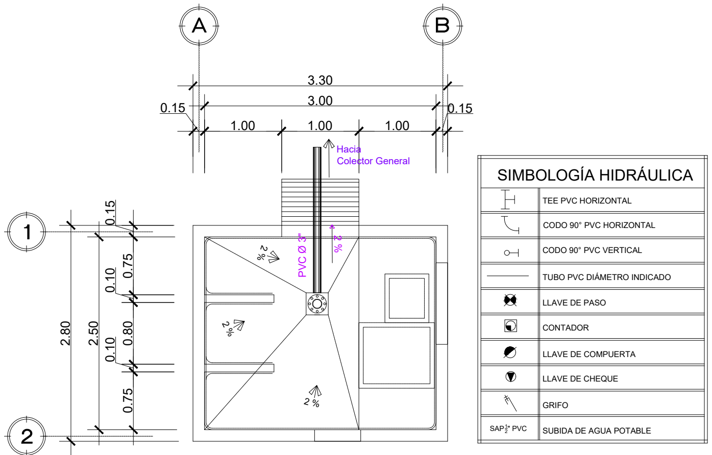
Figura 27: Planta hidráulica del centro de acopio propuesto | Crédito: equipo consultor.
