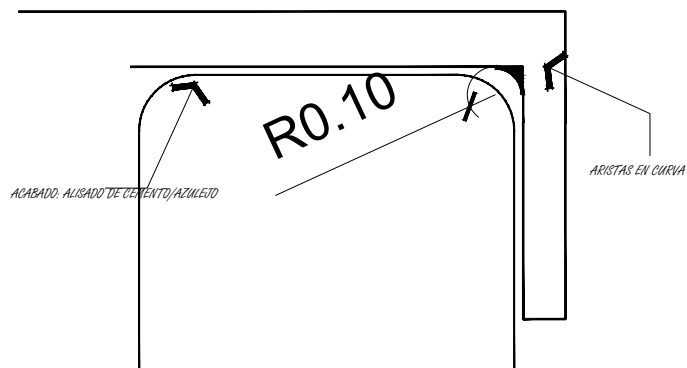
Figura 29: Detalle arista del centro de acopio propuesto, énfasis en curvas, (escala: 125) | Crédito: equipo consultor.
