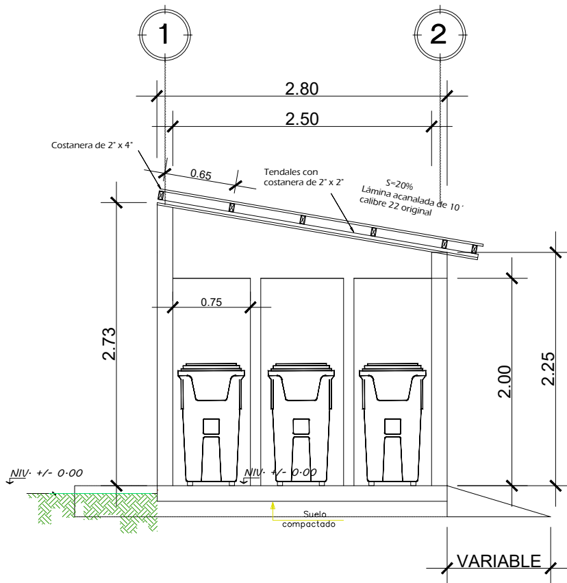
Figura 29: Sección transversal del centro de acopio propuesto | Crédito: equipo consultor.
