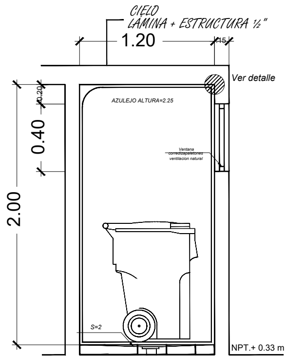
Figura 28: Detalle arista del centro de acopio propuesto (escala: 125) | Crédito: equipo consultor.
