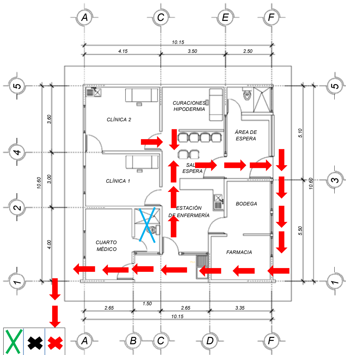
01 PLANTA ARQUITECTÓNICA PRIMER NIVEL. ESC.: 1:125
