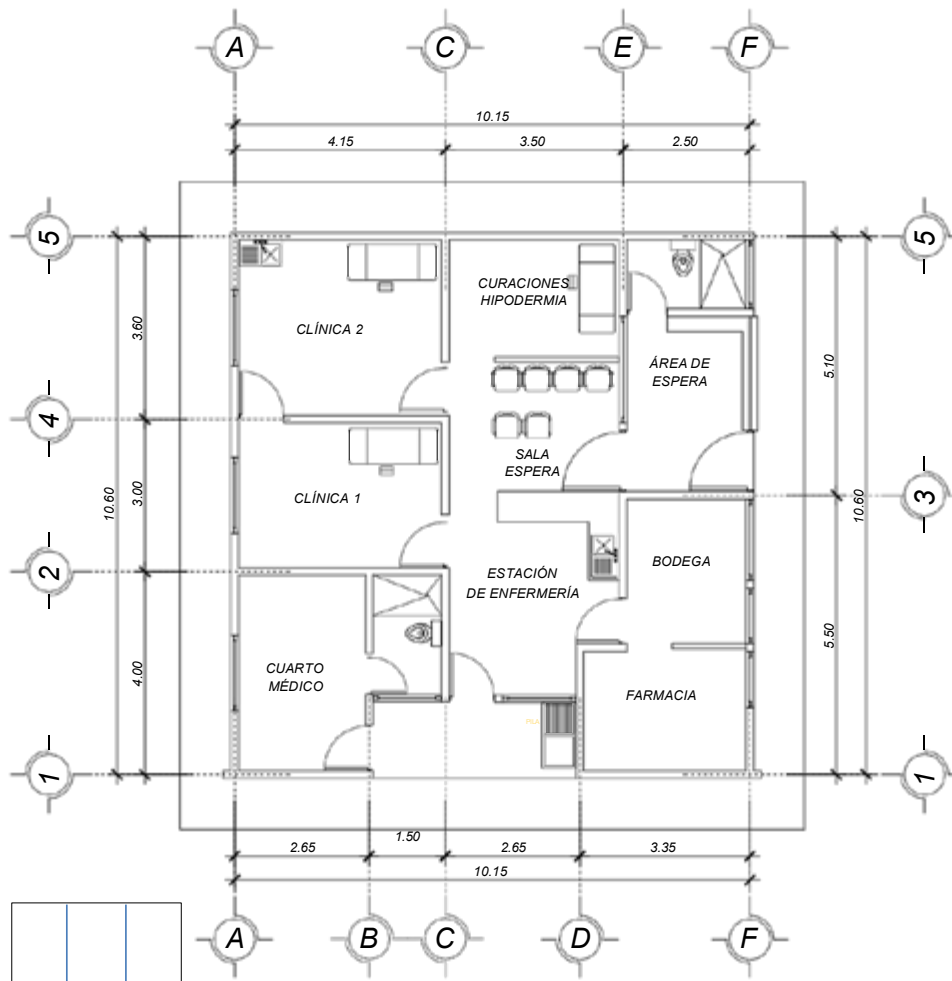
01 PLANTA ARQUITECTÓNICA PRIMER NIVEL. ESC.: 1:125
