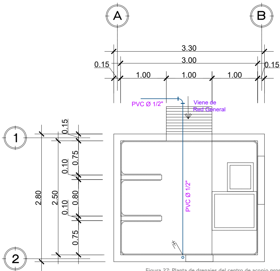
Figura 27: Planta de drenajes del centro de acopio propuesto | Crédito: equipo consultor.
