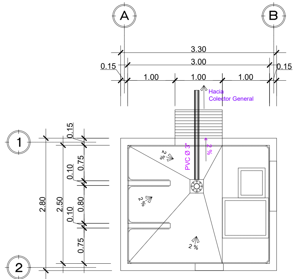
Figura 28: Planta hidráulica del centro de acopio propuesto | Crédito: equipo consultor.
