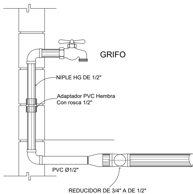
Figura 34: Detalle de grifos del centro de acopio propuesto (escala 1/20) | Crédito: equipo consultor.
