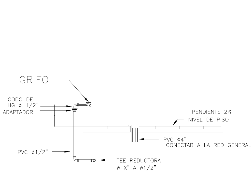
Figura 33: Alzado para grifo y salida de drenaje del centro de acopio propuesto | Crédito: equipo consultor.
