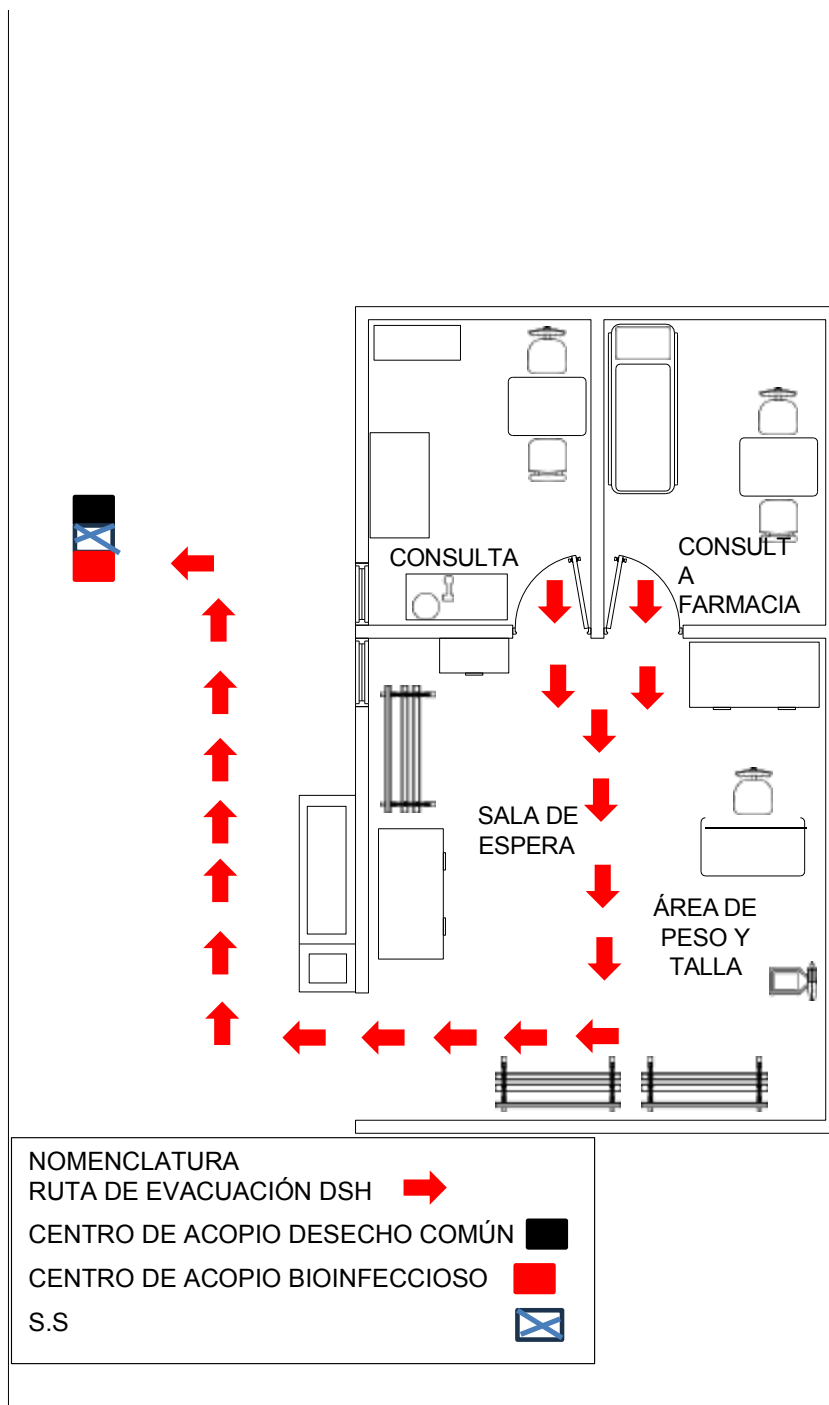
Figura 60: Plano con ruta de evacuación del Centro comunitario de salud Tujolom | Crédito: equipo consultor.
