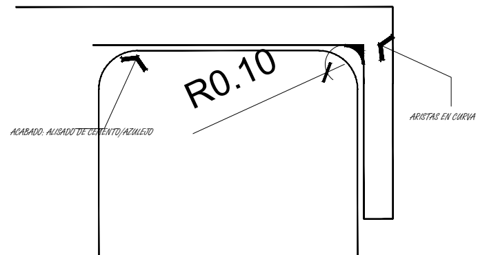
Figura 30 y figura 31: Detalle arista del centro de acopio propuesto (escala: 125) y detalle arista del centro de acopio propuesto, énfasis en curvas, (escala: 125) | Crédito: equipo consultor | Crédito: equipo consultor.
