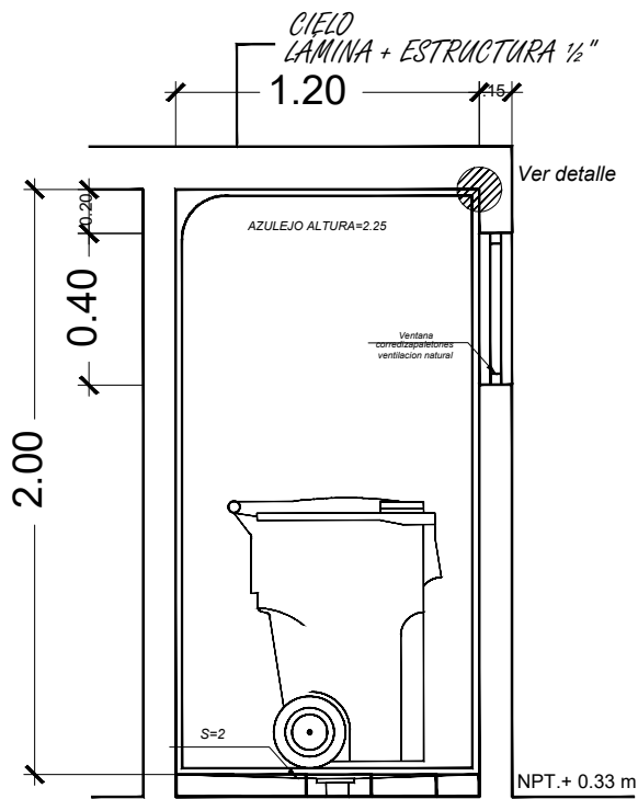
Figura 30 y figura 31: Detalle arista del centro de acopio propuesto (escala: 125) y detalle arista del centro de acopio propuesto, énfasis en curvas, (escala: 125) | Crédito: equipo consultor | Crédito: equipo consultor.
