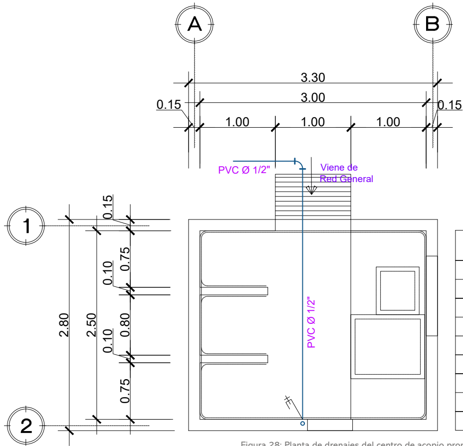
Figura 28: Planta de drenajes del centro de acopio propuesto | Crédito: equipo consultor.
